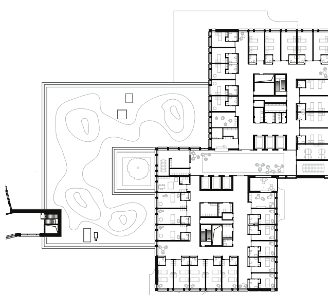
Grundriss 2. Obergeschoss .
